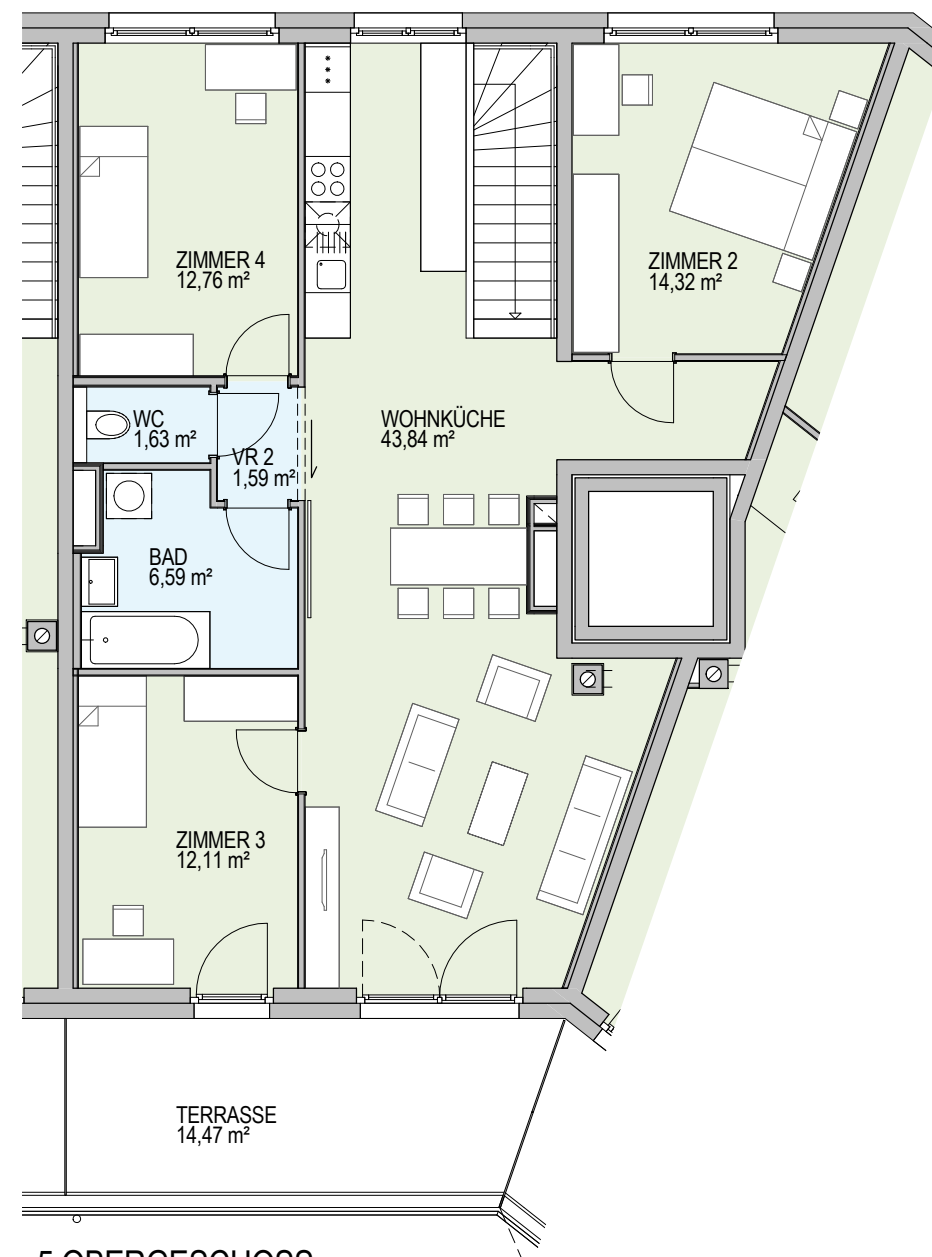
5.OBERGESCHOSS
