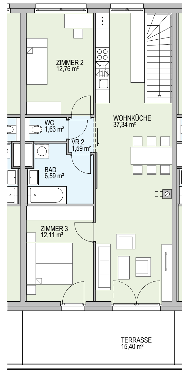
5.OBERGESCHOSS
