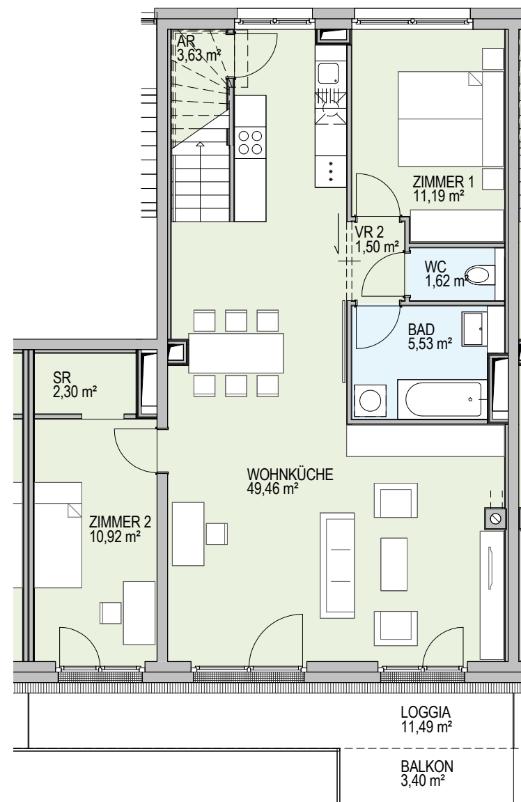
3.OBERGESCHOSS
