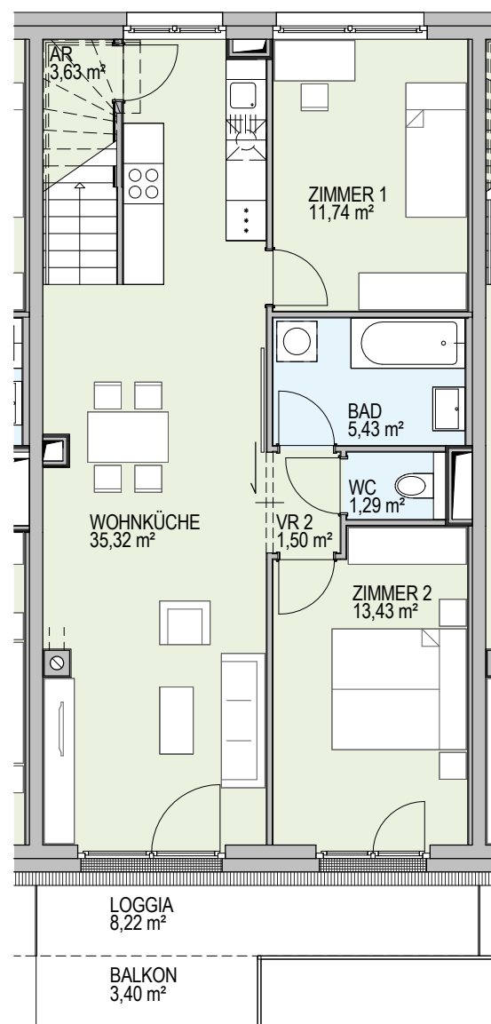
3.OBERGESCHOSS
